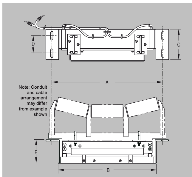
MSI dimensions
